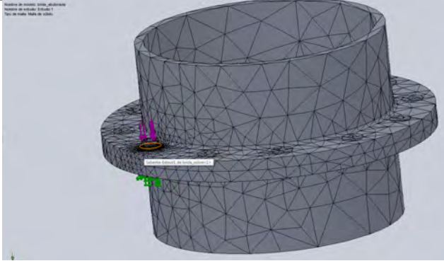
Fig. N°8 Mallado con control adaptativo, fuente propia.
