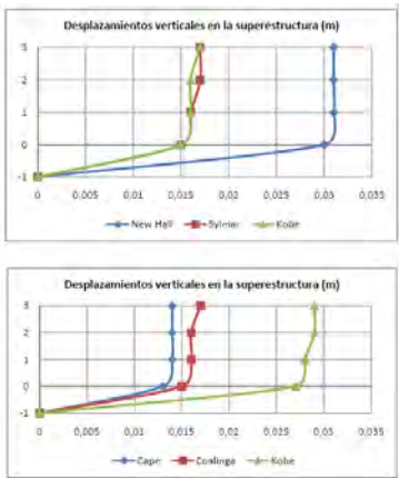
Figura 14 Desplazamientos verticales en la superestructura
