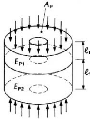
Fig. N°4. Simplificación del modelo para el cálculo de la rigidez. Fuente ídem.
