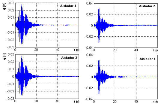
Figura 4 Desplazamientos dirección vertical. Terremoto New Hall
