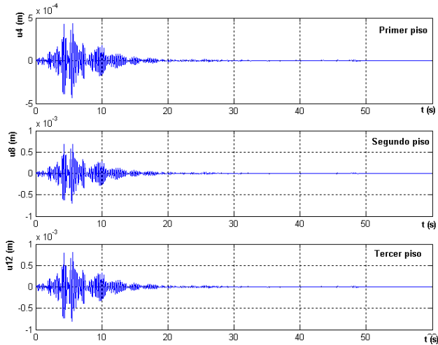
Figura 12 Desplazamientos verticales en la superestructura. Registro sísmico de New Hall. Fire Station (1994).
