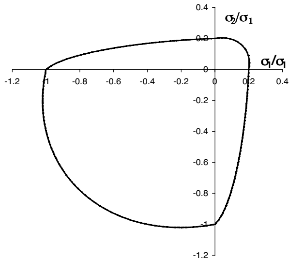
Figura 2: Curva umbral de daño en el plano \tilde{\sigma}_1 - \tilde{\sigma}_2 , para un material con isotropía elástica.
