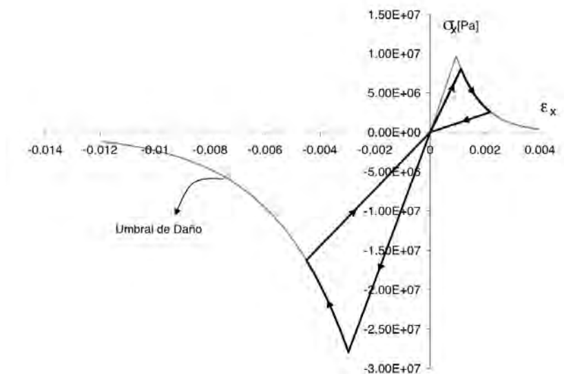
Figura 4: Curvas tensión-deformación para historias de carga uniaxiales con reversión del sentido de la carga, \eta = 0,25 \xi = 0,25
