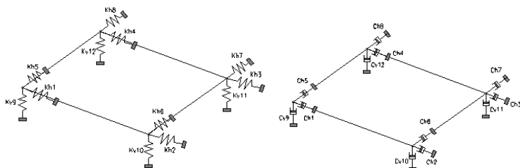
Figura 2 Rigidez y amortiguamiento en la posición de cada aislador y amortiguador viscoso
