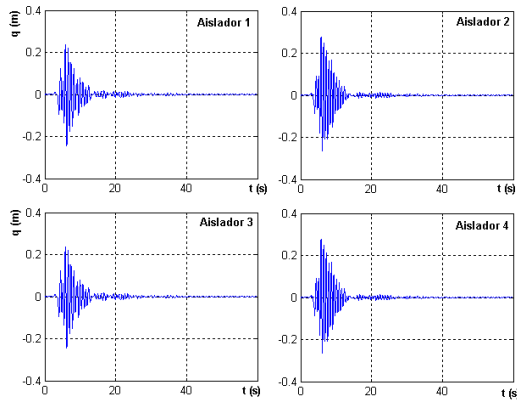
Figura 3 Desplazamientos en dirección X. Terremoto New Hall
