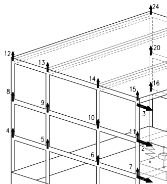
Figura 6 Grados de libertad admitidos en la superestructura
