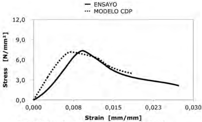
Figura 8: Tensión-Deformación Pila de Mampostería PL290.
