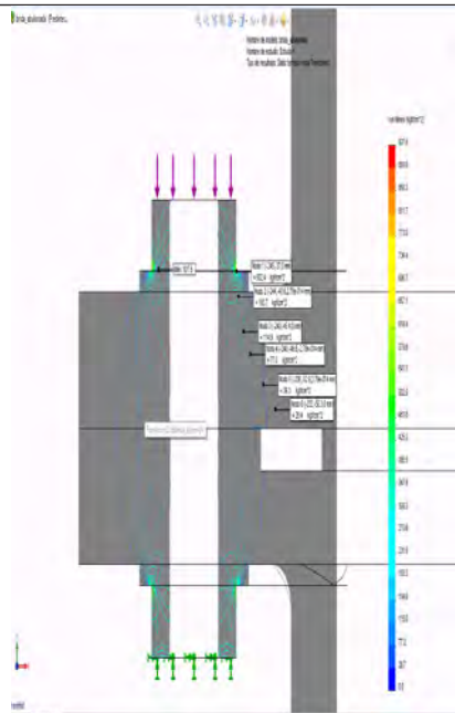
Fig. N°11 Líneas de isotensión en el modelo de junta mediante Solver "Cosmos". Fuente propia.
